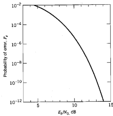
Figure 14: Bit Error Rate (BER)
